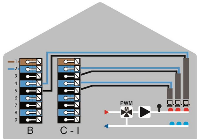
Actuadores para zonas de aquecimento
