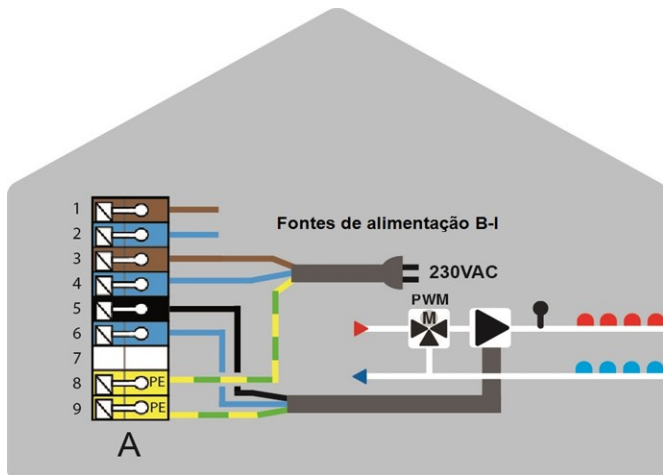
Conexões á bomba de circuito de aquecimento
