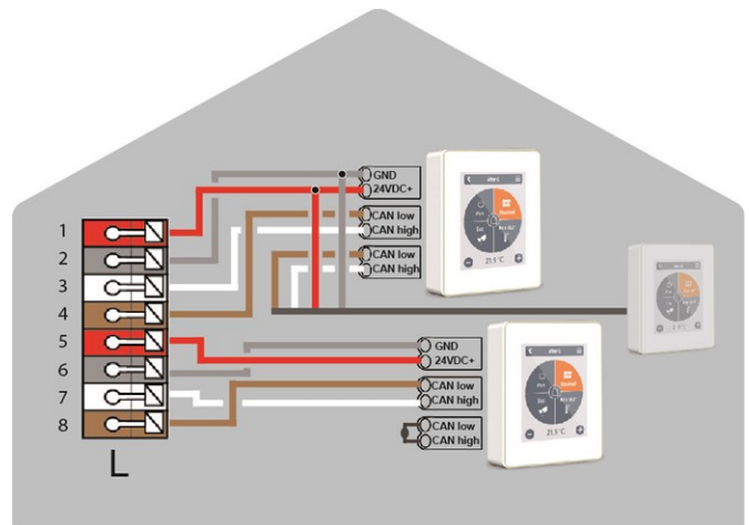
Controlador °CALEON em CAN bus em rede privada
