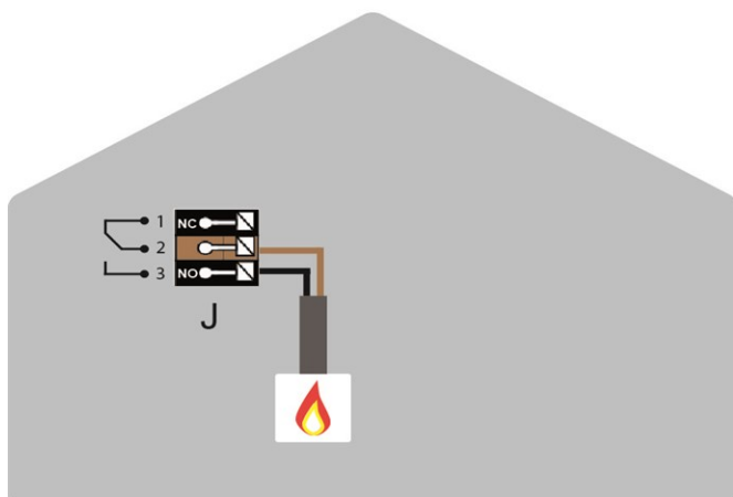
Contactos secos para funções adicionais
