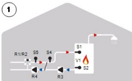
Mischerregelung
