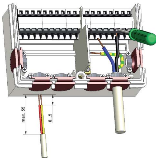
Abb.3.2.1
