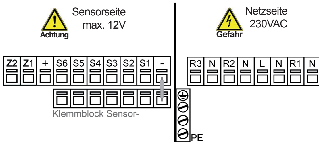
Abb. 3.3.2 „Mit Zirkulationspumpe“
