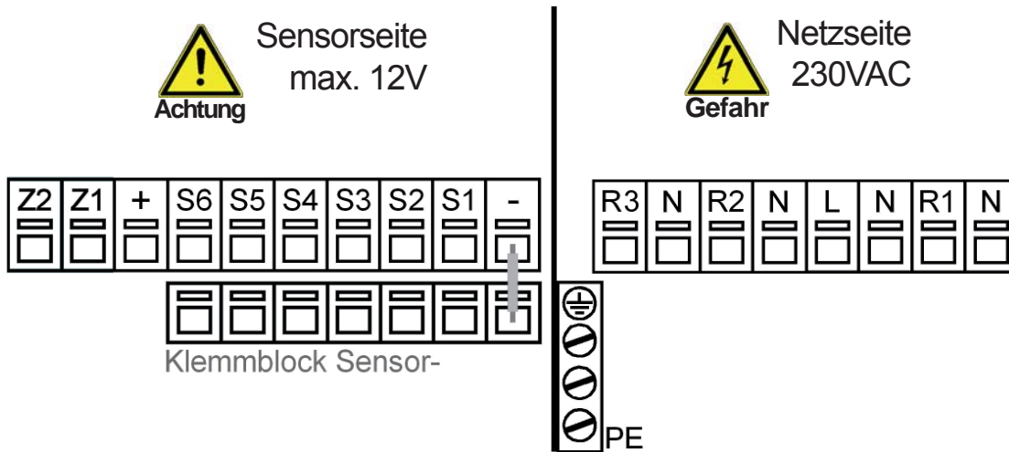
Abb. 3.3.1 „Ohne Zirkulationspumpe“
